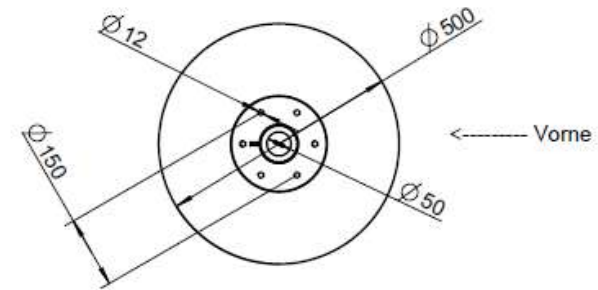
SCHNITT A-A
